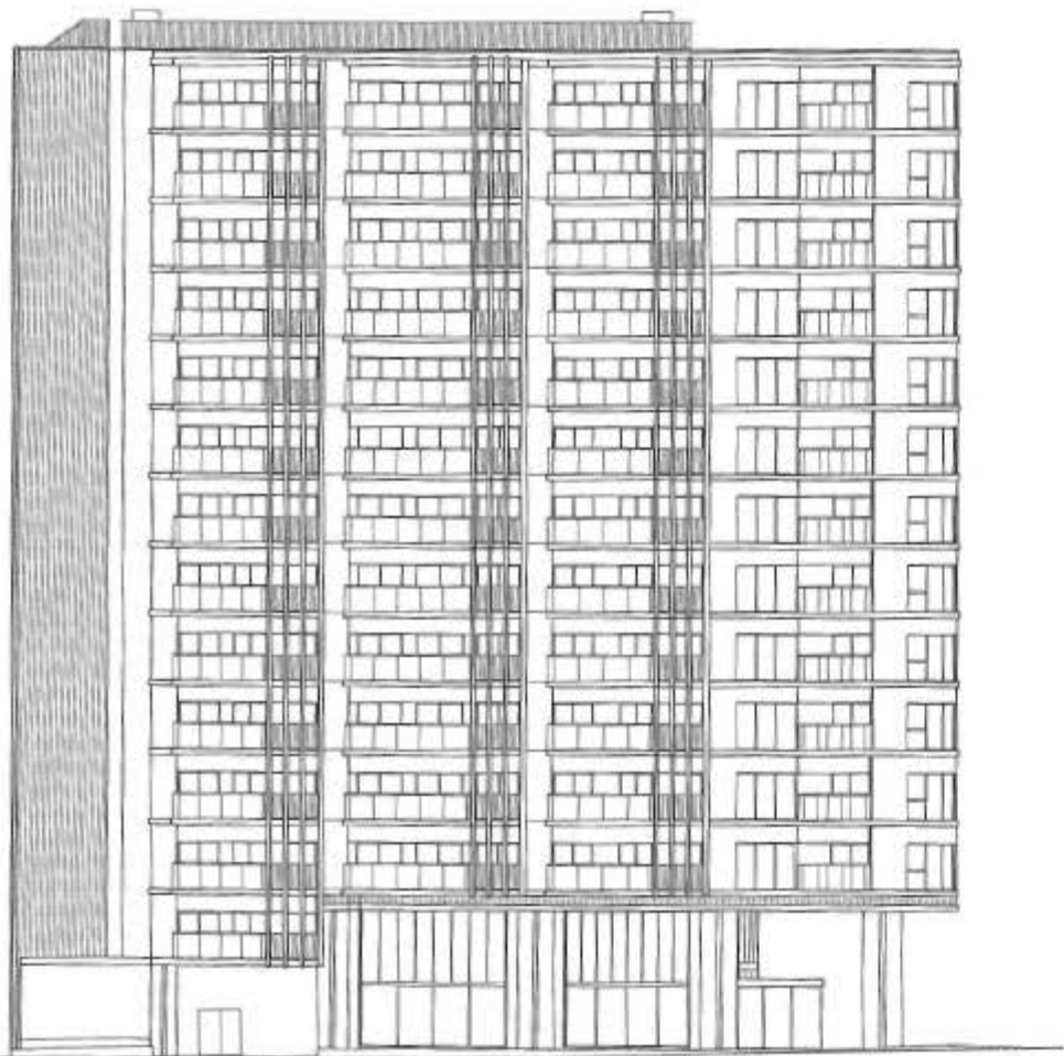
南東側立面圖
